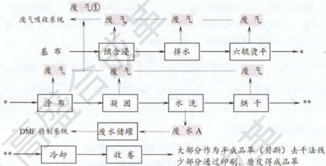
图 4.1-1 PU 合成革湿法生产线工艺流程图
