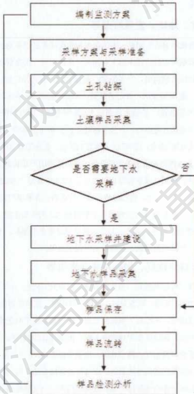
图1.3-2工作程序
