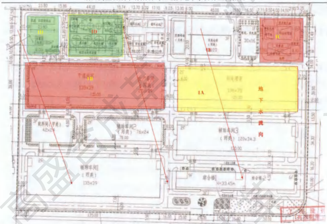
图5.2-1浙江高盛合成革有限公司疑似污染区域图
