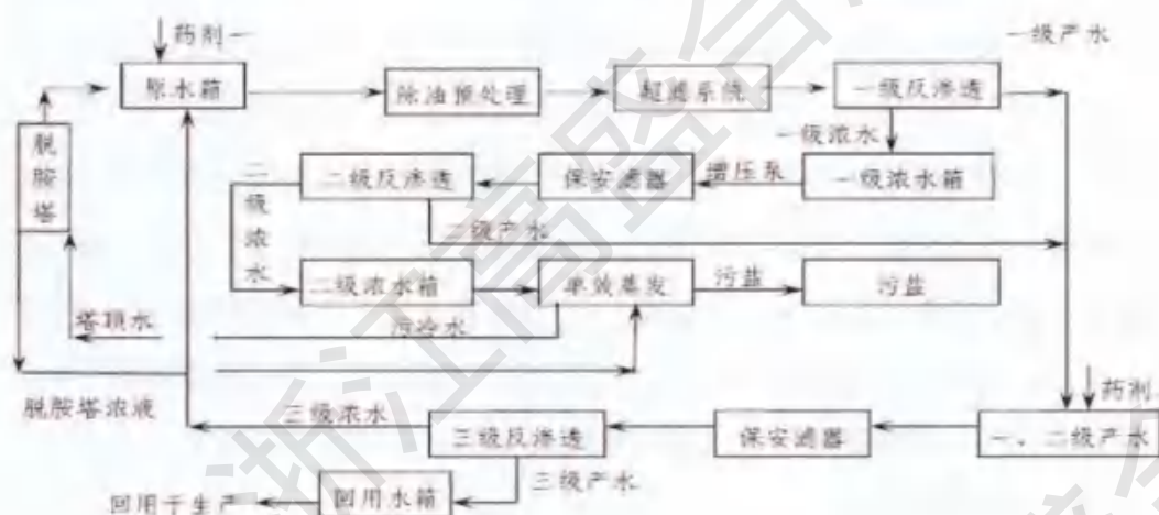
图 4.1-3 膜处理系统
