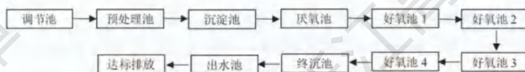
图 4.1-4 生化污水处理装置工艺流程图
