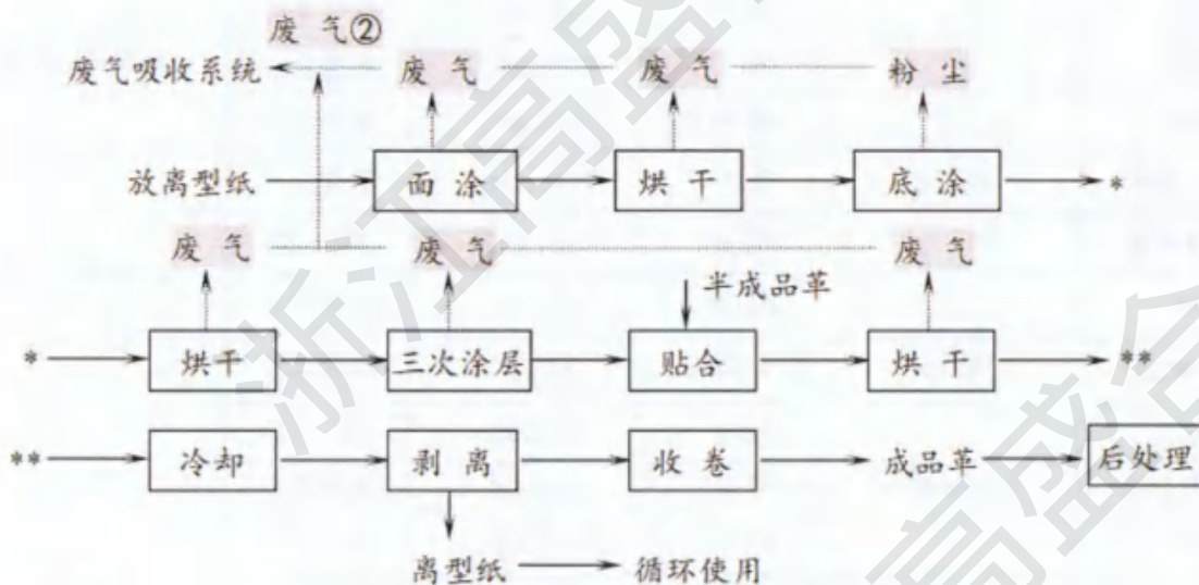
图 4.1-2 PU 革干法生产线工艺流程
